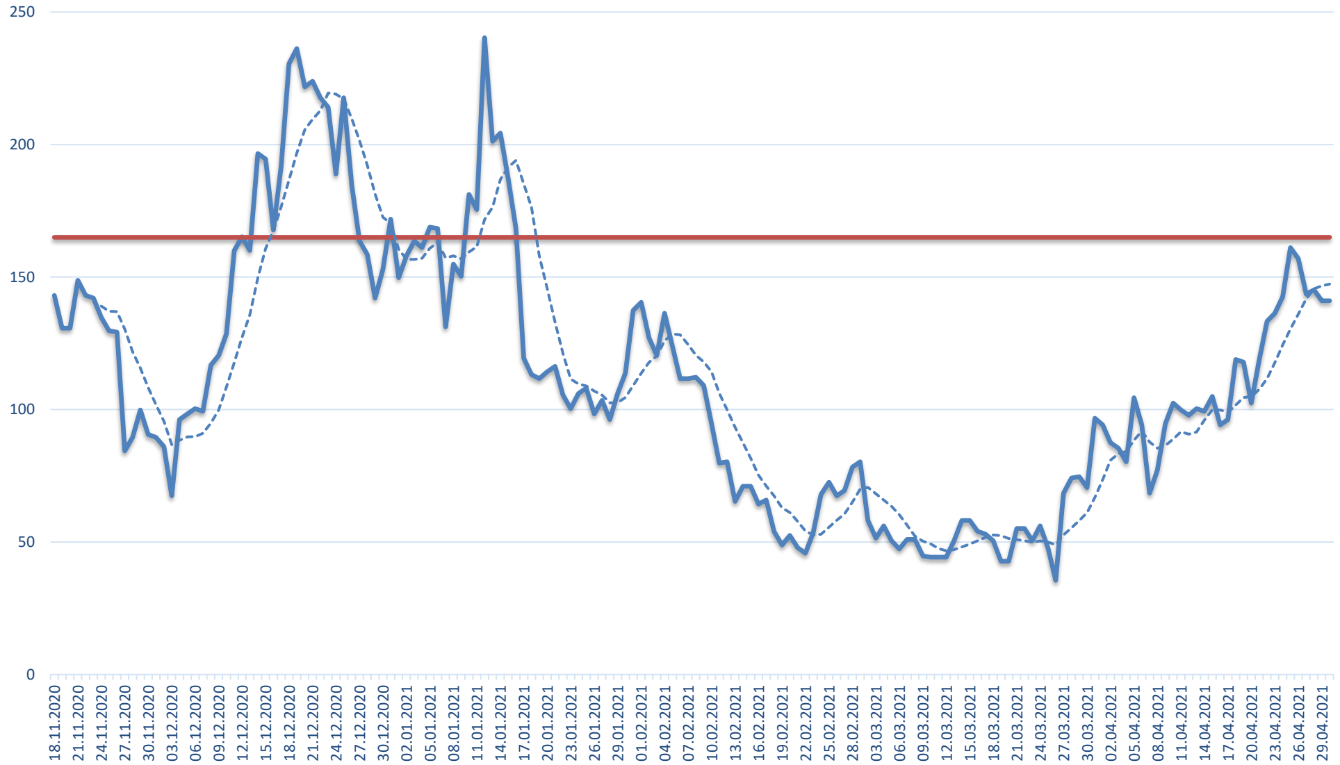
RKI-7-Tage-Inzidenz für den Landkreis Saarlouis gemäß der Daten von www.rki.de/inzidenzen vom 30.04.2021, 09:00 Uhr
